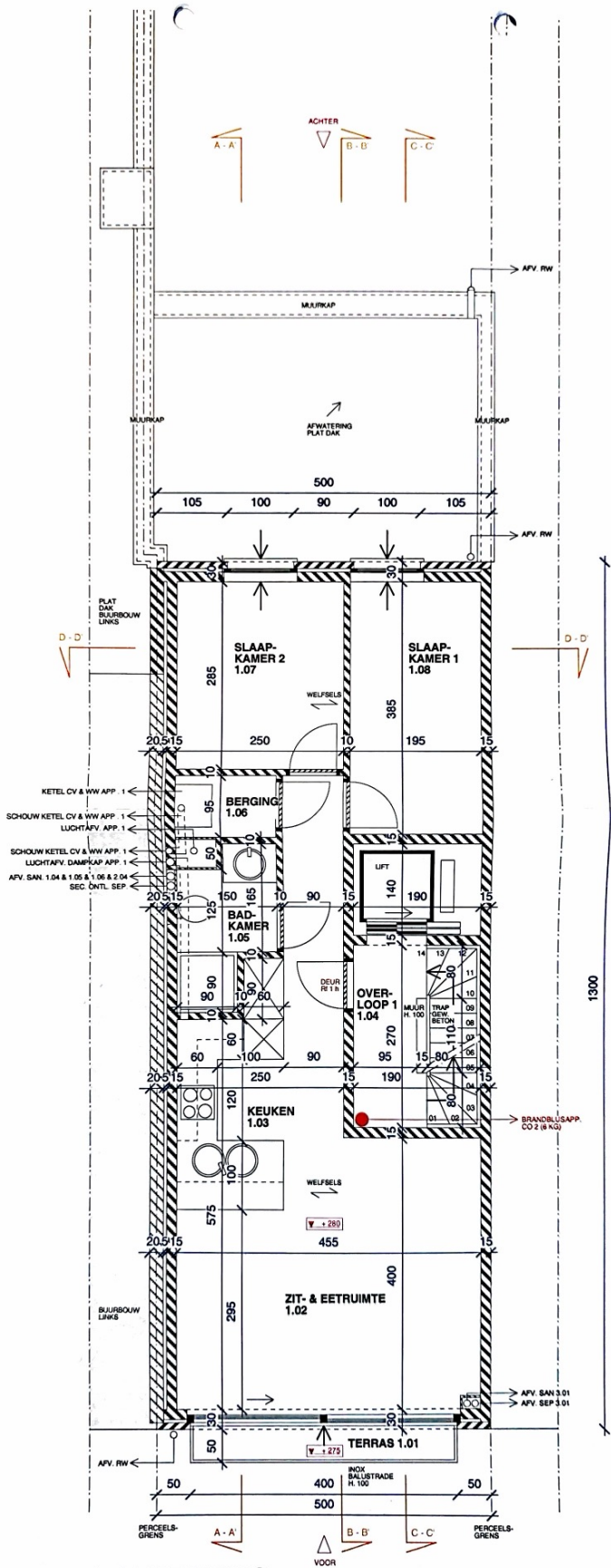
1e VERDIEPING
