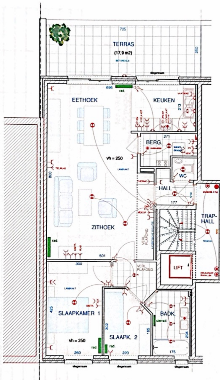
VERDIEPING 1 type 1.A
