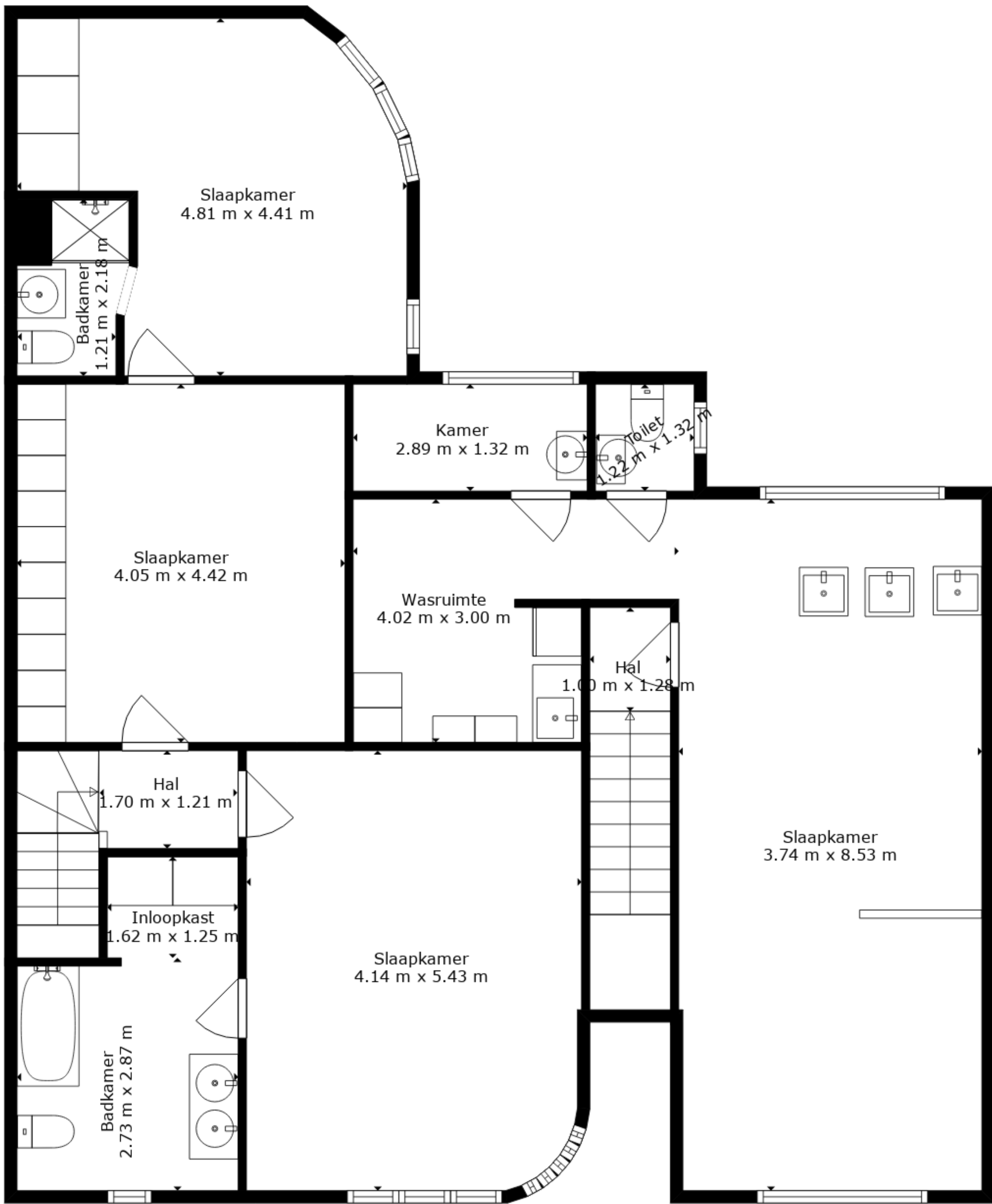
3. Verdieping
