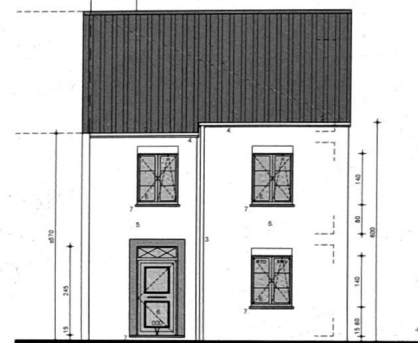
VOORGEVEL
