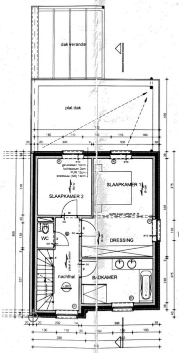
VERDIEPING
