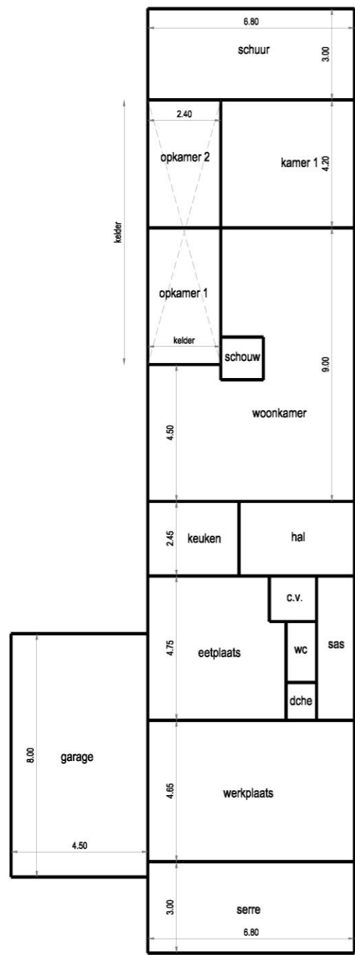
GELIJKVLOERS
