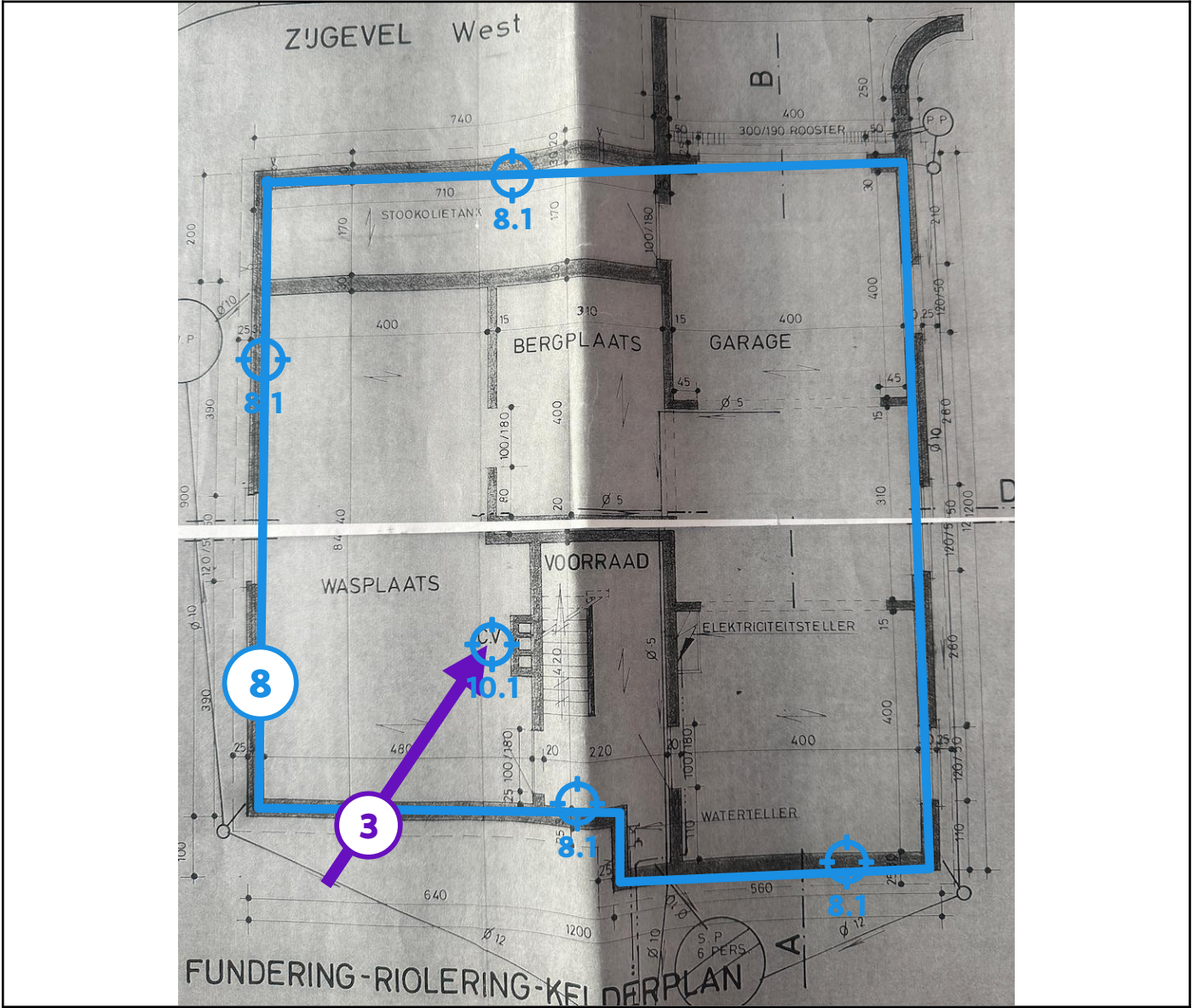
Legende van plan 1.1: Kelder
