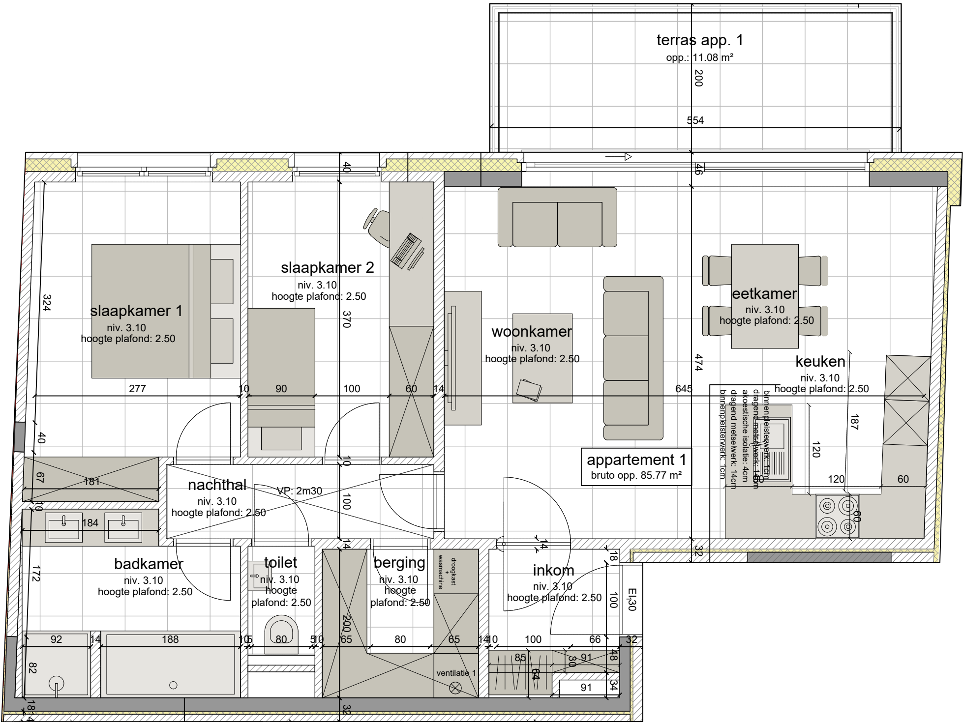
Plan inrichting - schaal 1/50
