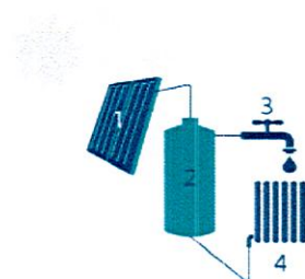
1 zonnecollector 2 opslagvat 3 sanitair warm water 4 ruimteverwarming 4 zonnecollector 5 opslagvat 6 sanitair warm water 7 ruimteverwarming
