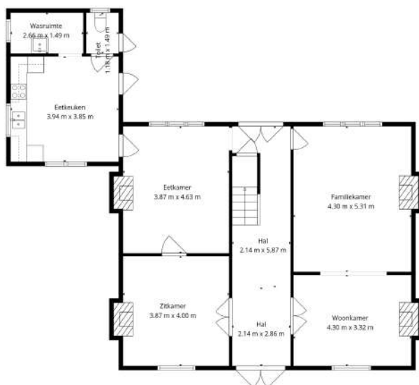
1e Verdieping
