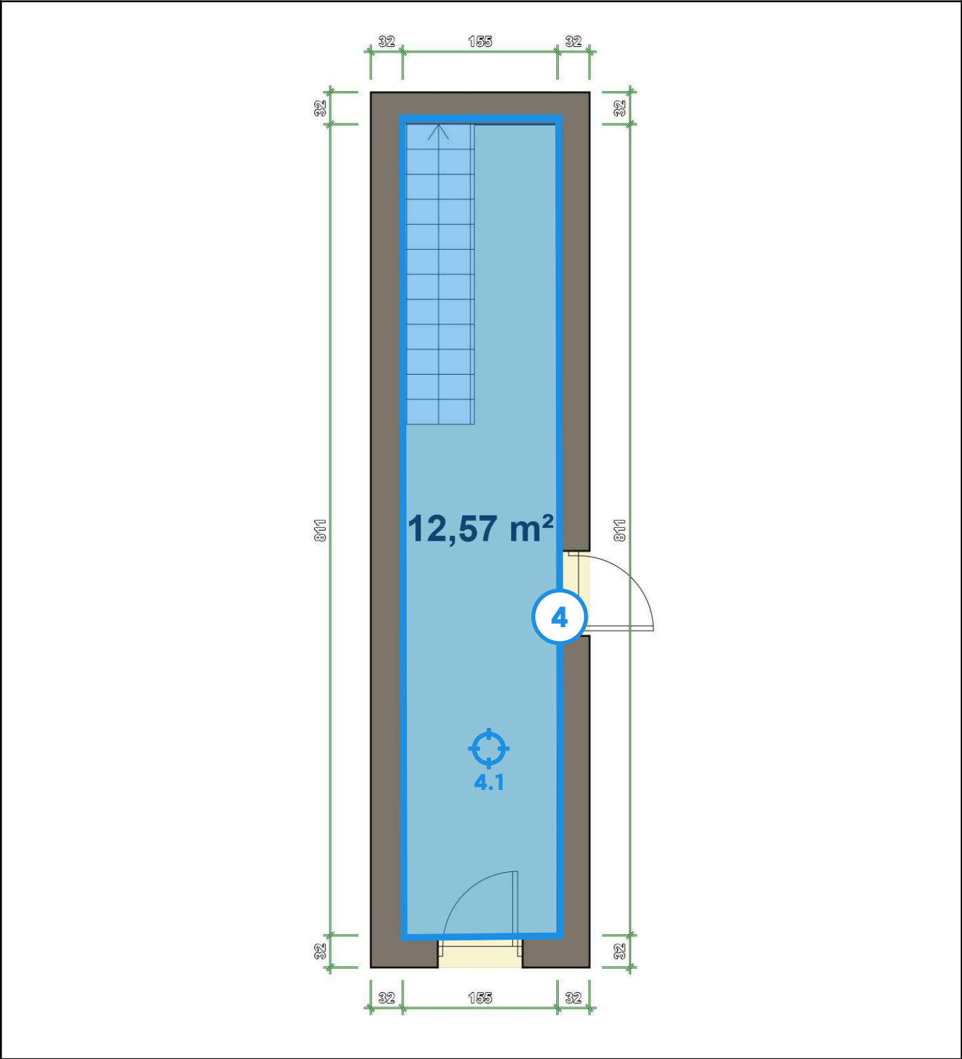
Legende van plan 1.3: Traphal gelijkvloers plafond
