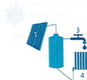
1 Zonnecollector | 2 Opslagvat zonneboiler | 3 Tap 4 Sanitair warm water Als toelement voor ruimteverwarming (optioneel) radiator
