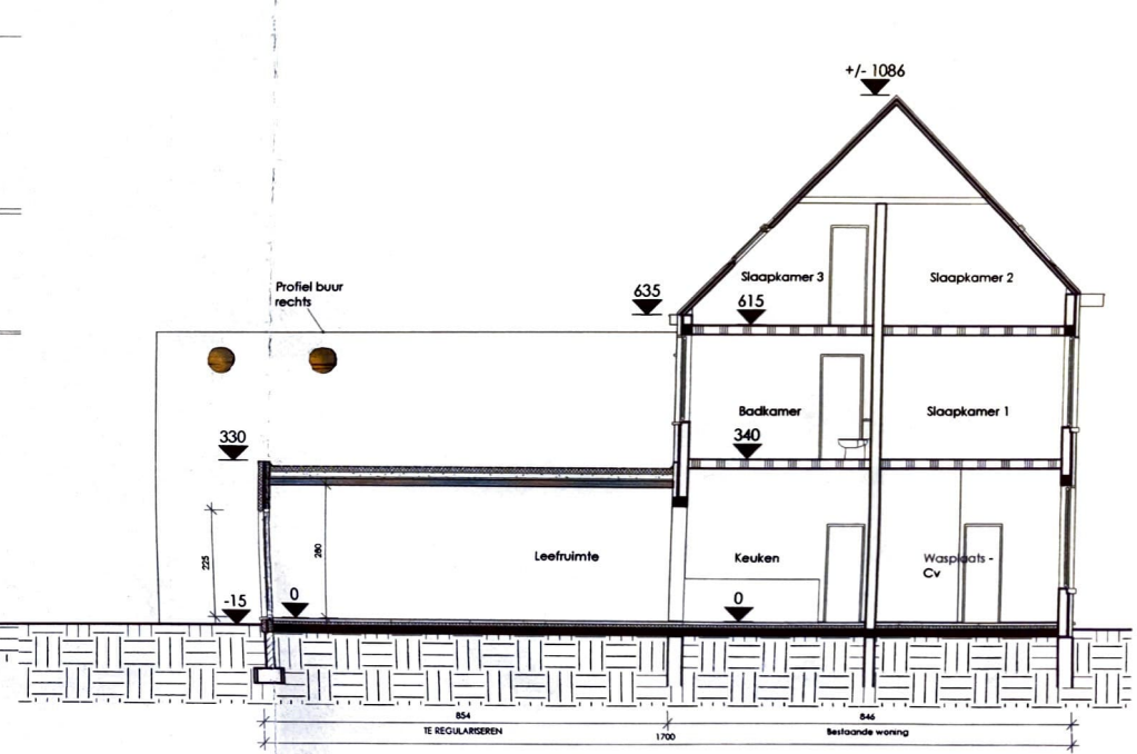
Doorsnede AA'
