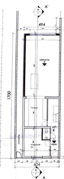
Gelijkvloers
