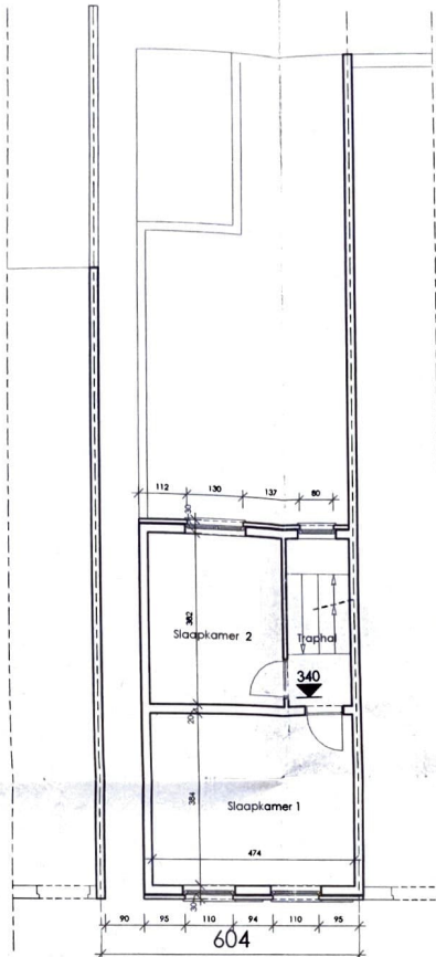
Verdieping 1
