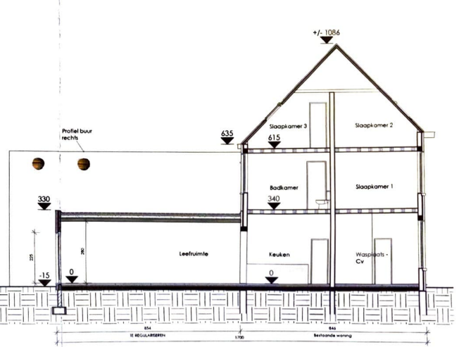
Doorsnede AA'
