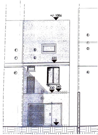
Achtergevel
