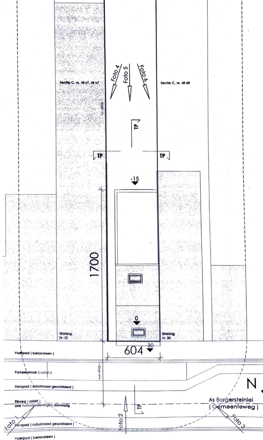
Inplantingsplan ( schaal 1/250 )
