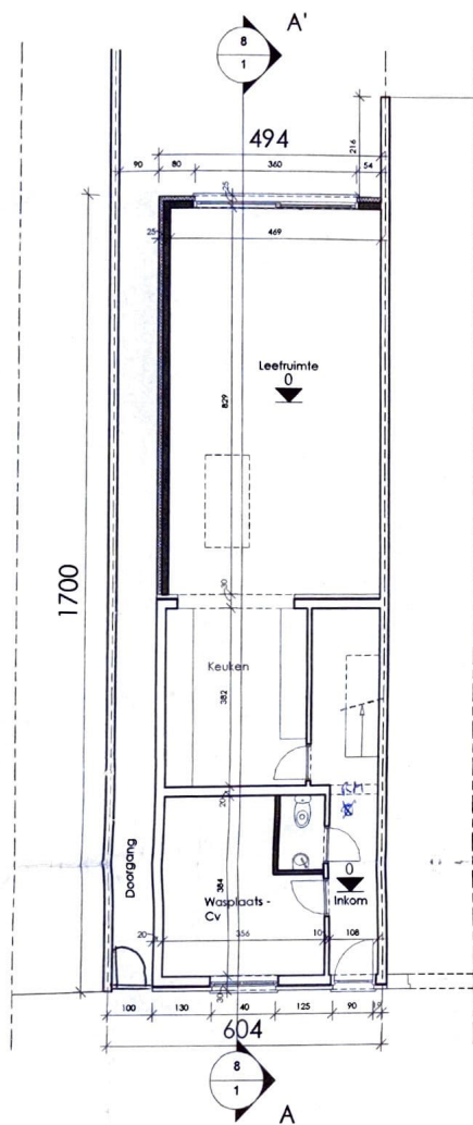
Gelijkvloers
