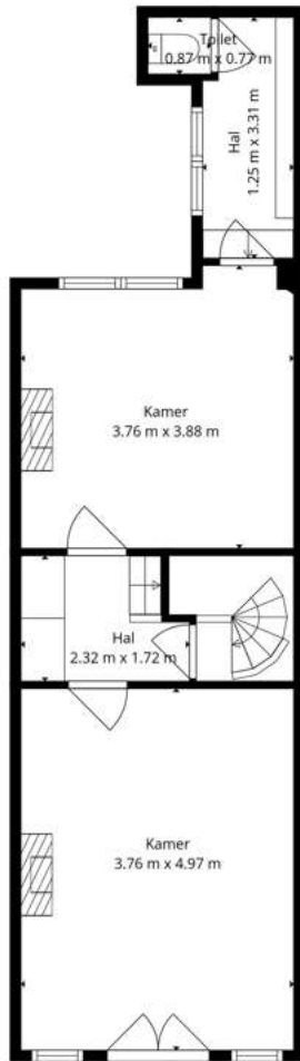
1ste Verdieping
