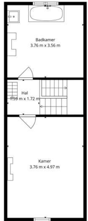
3ste Verdieping
