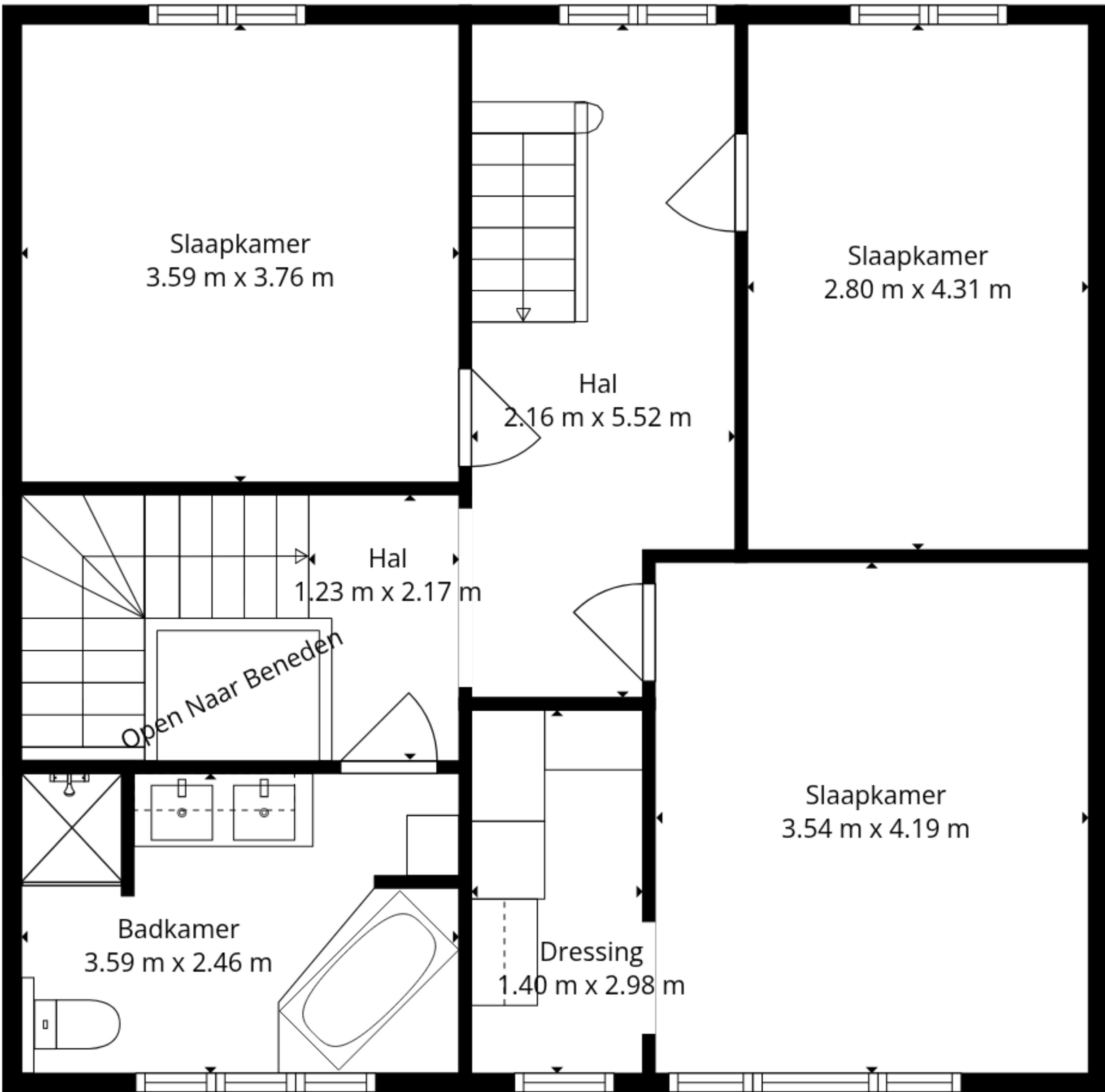
1e Verdieping
