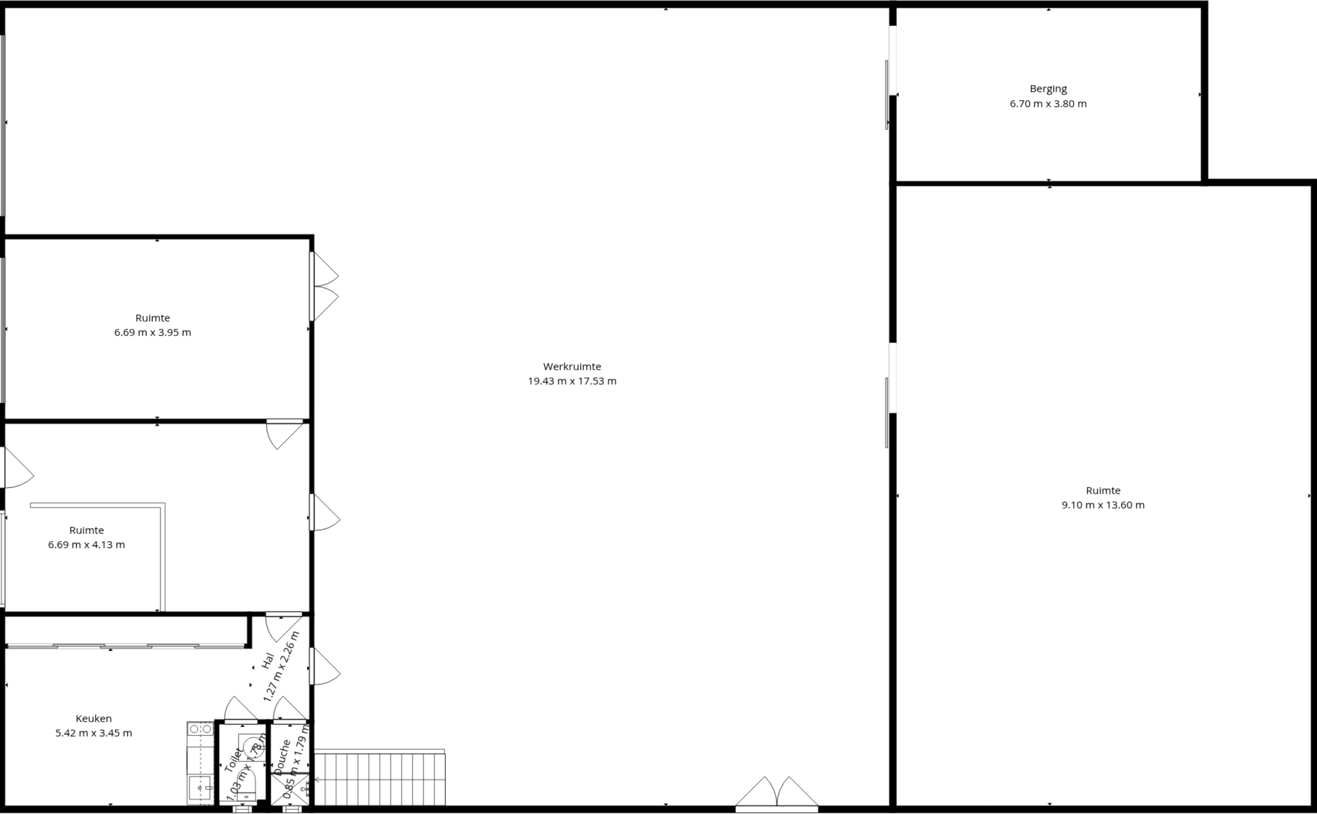
1e Verdieping
