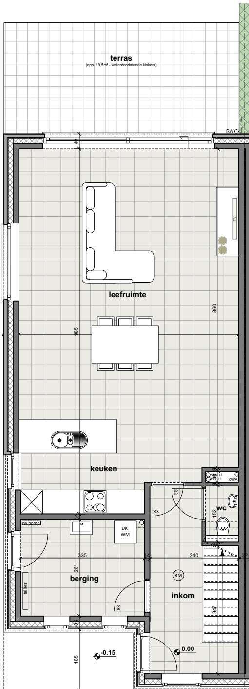
Gelijkvloers
