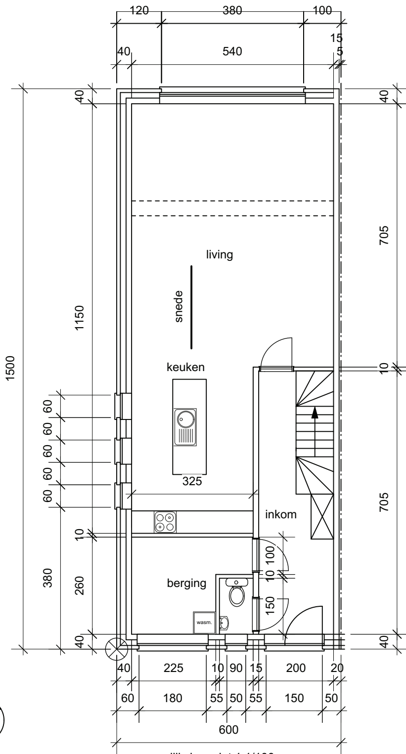
gelijkvloers lot 1 1/100
