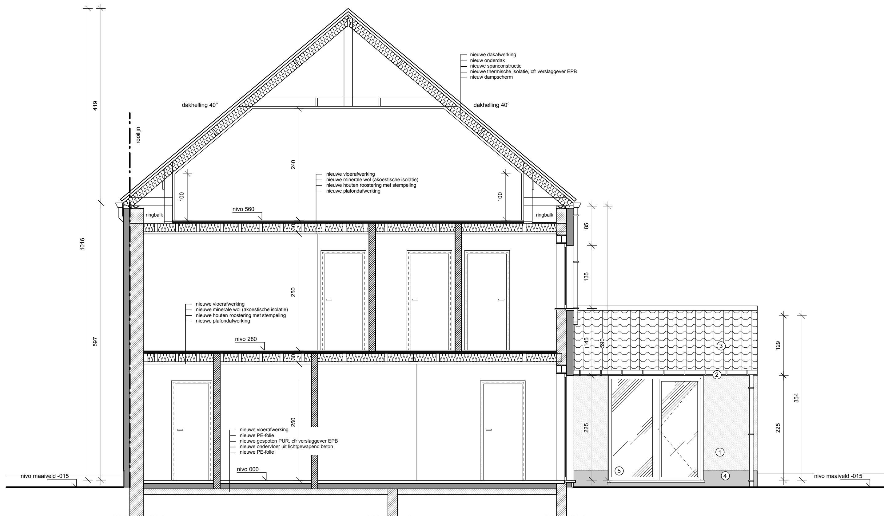
DOORSNEDE AA ontworpen toestand schaal 1/50
