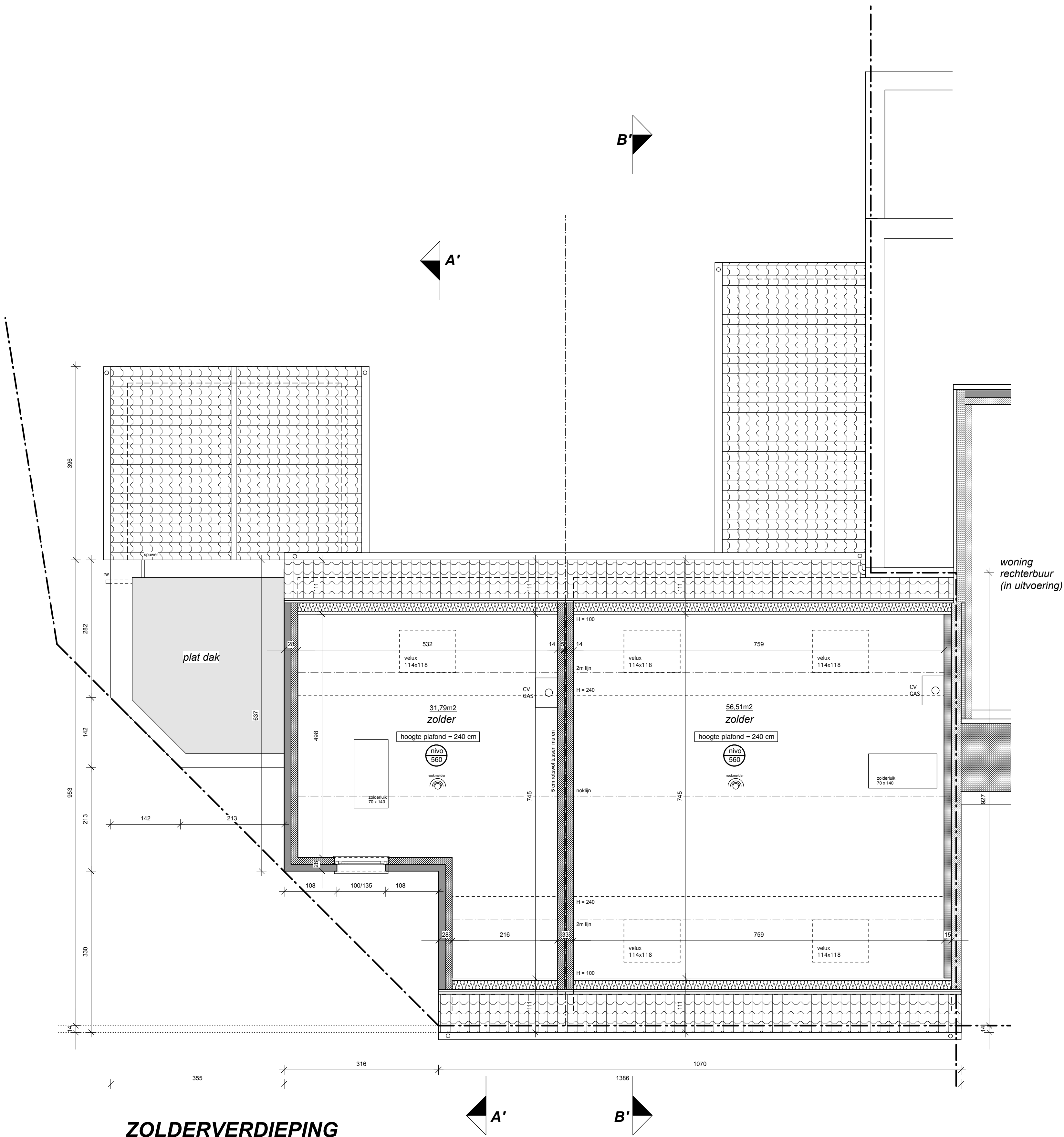
ZOLDERVERDIEPING ontworpen toestand schaal 1/50
