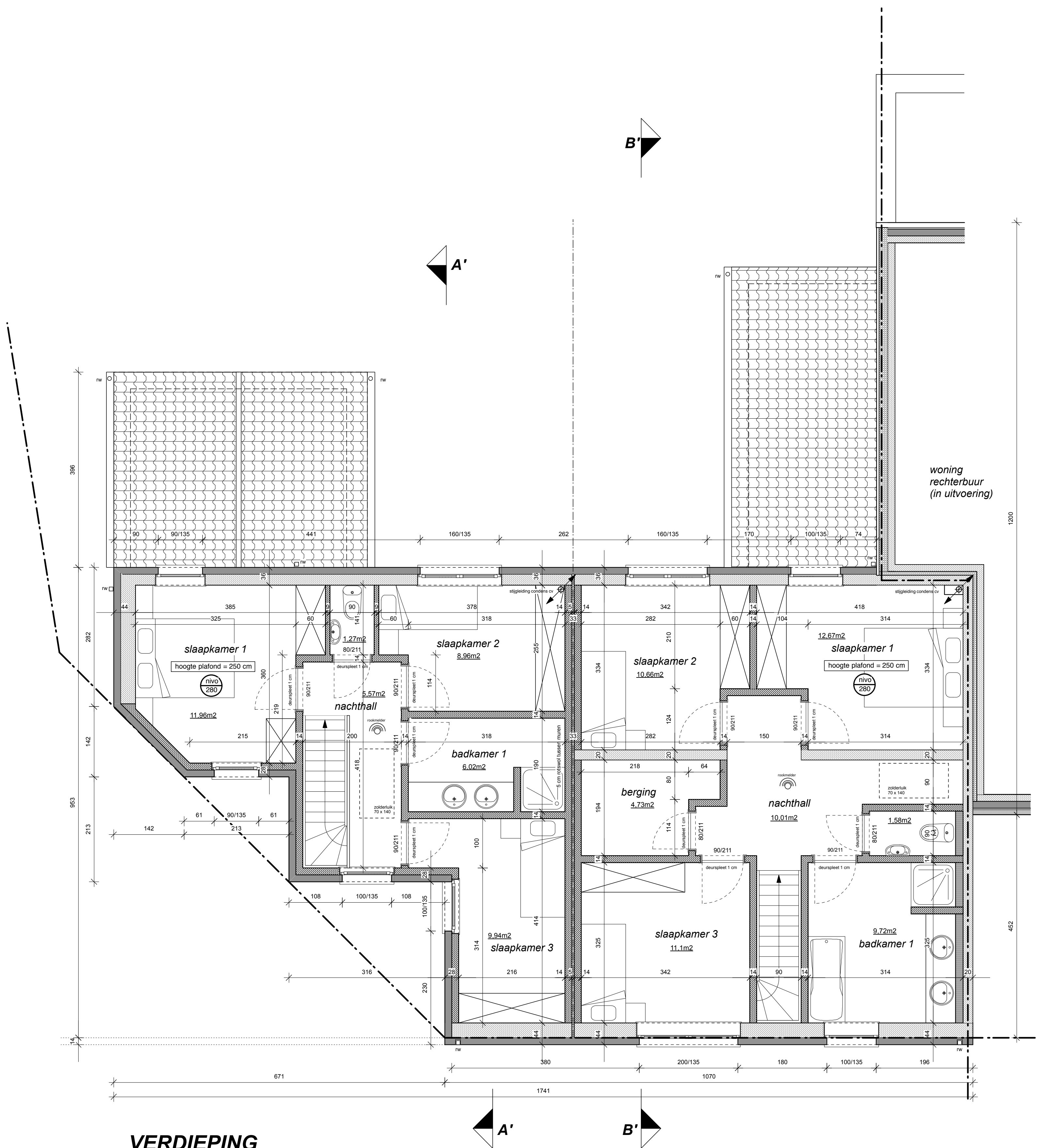
VERDIEPING ontworpen toestand schaal 1/50
