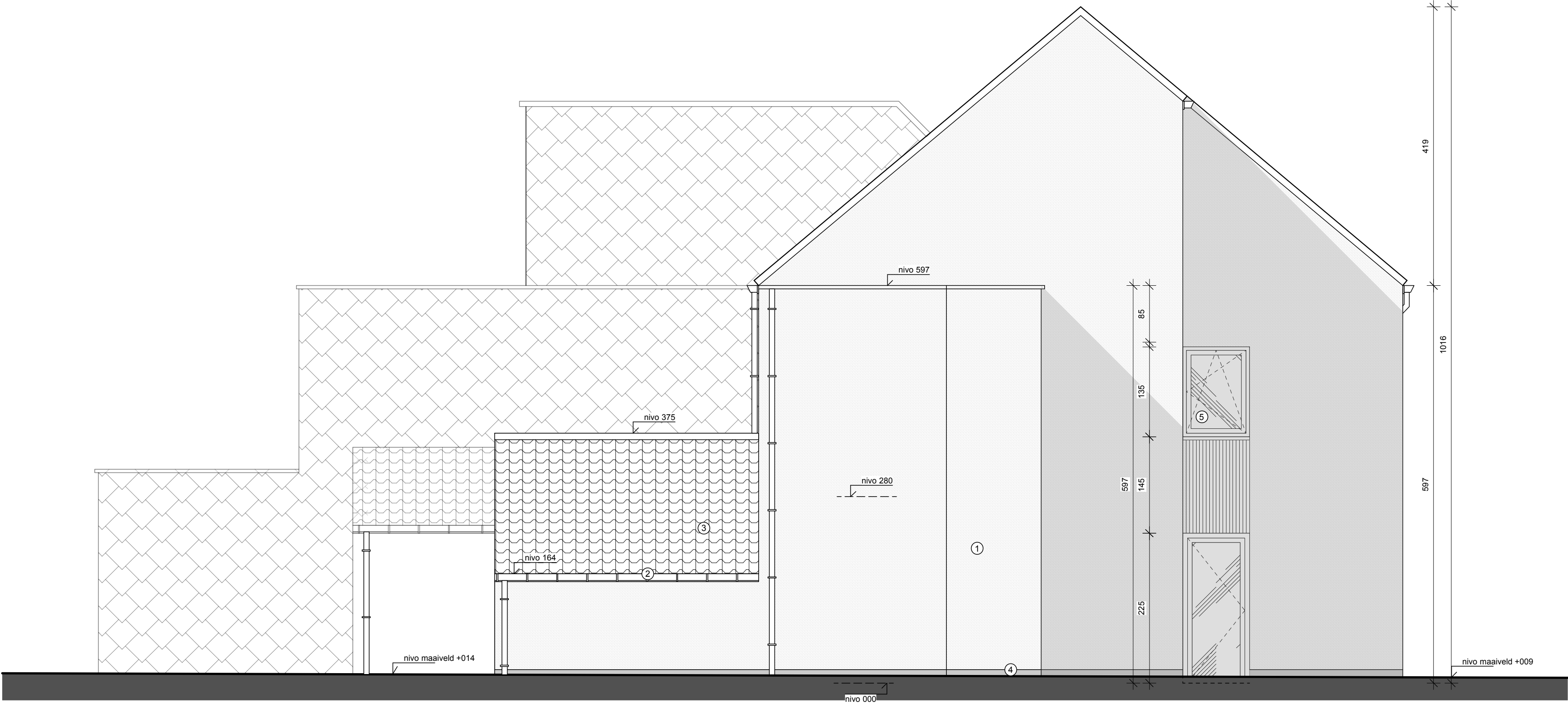
LINKERGEVEL ontworpen toestand schaal 1/50
