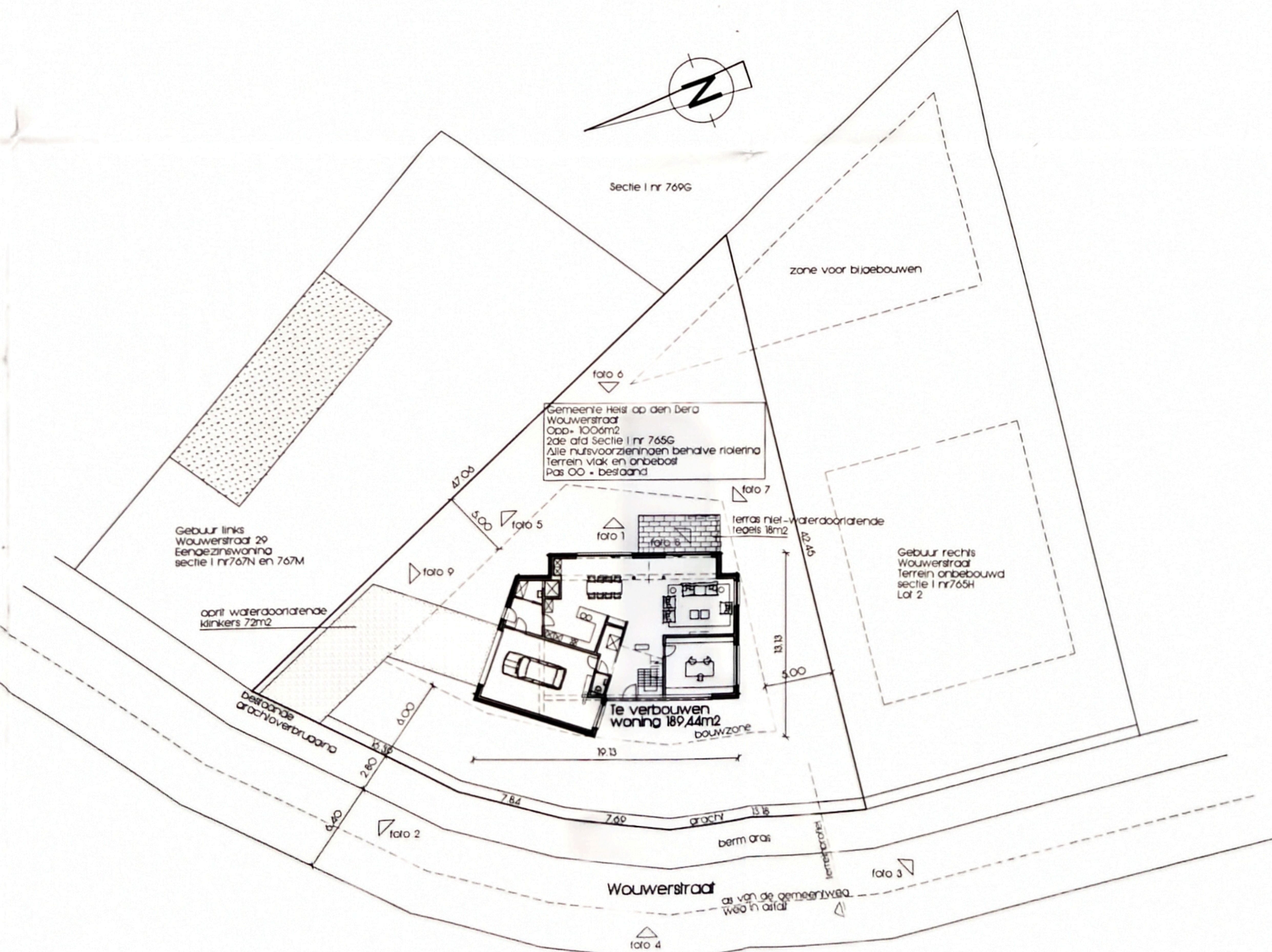
Inplantingsplan schaal 1/250
