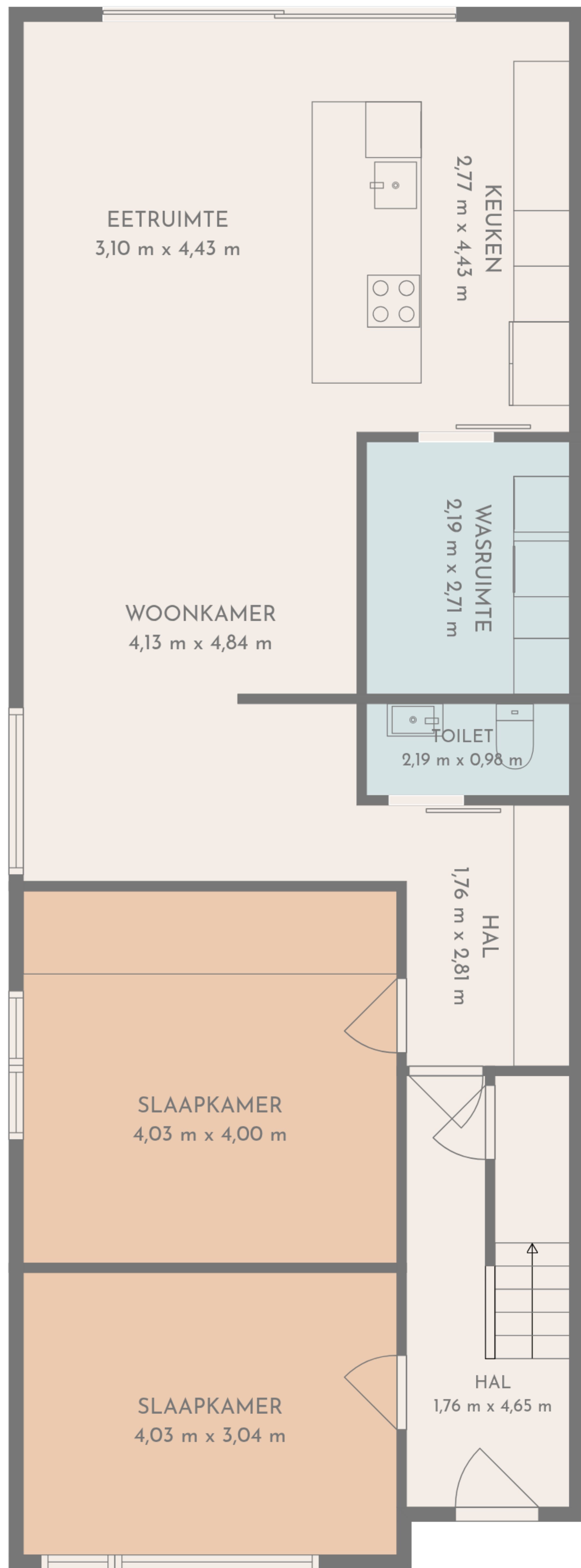
1e verdieping
