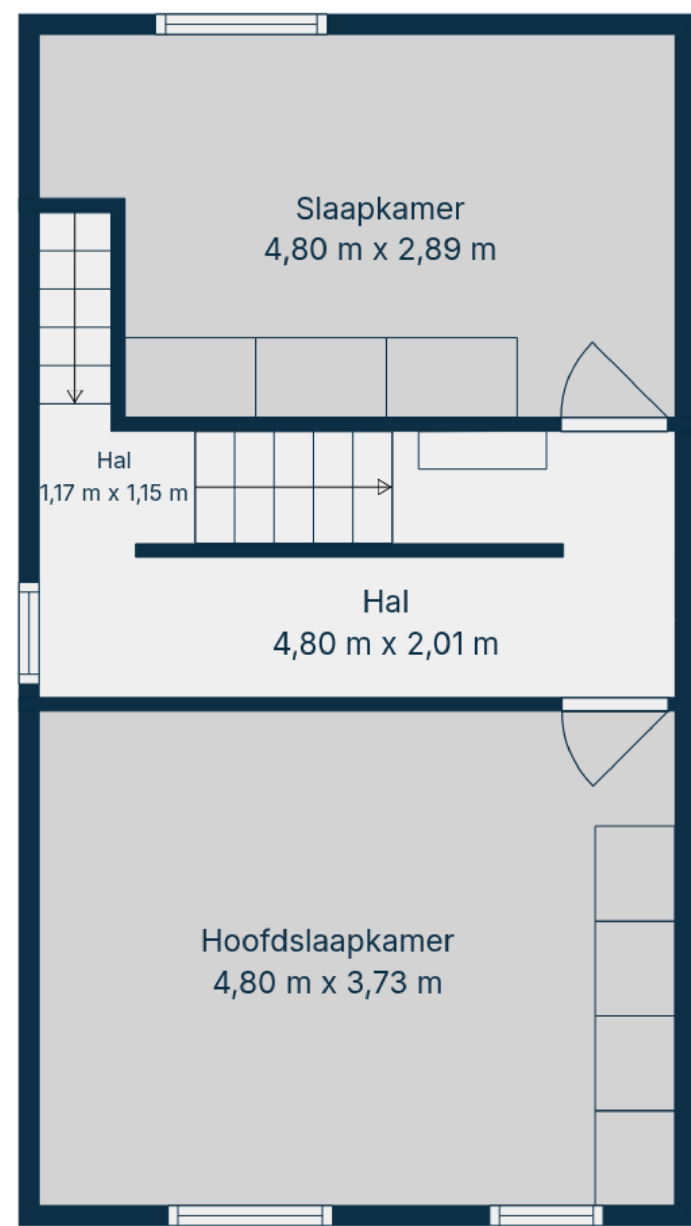
2e Verdieping
